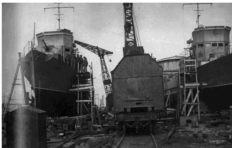
Постройка больших морских охотников проекта 122А
